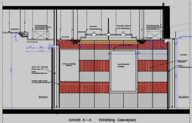
Schnitt A-A Windfang Seeplatz
